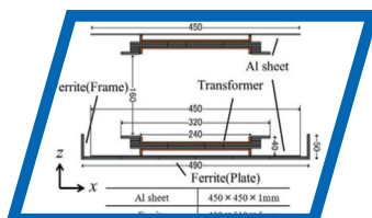
非接触供电变压器 Non-contact power supply transformer
