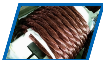
75kw电感 75kw inductance
